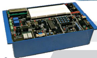
Microcontroller Trainer
